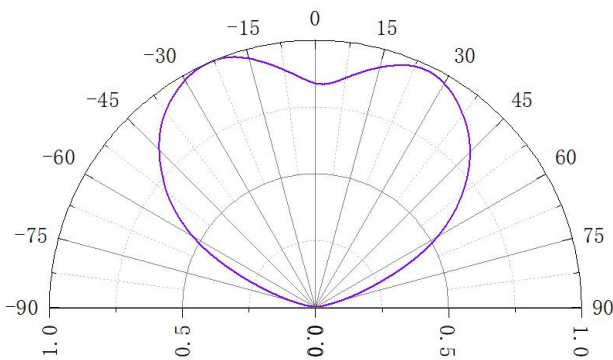
角度辐射特性曲线图
