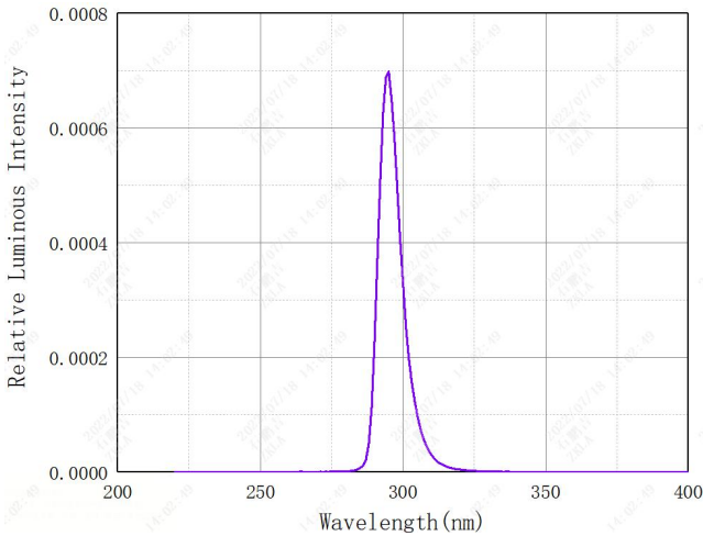
相对发光强度与波长关系曲线图
