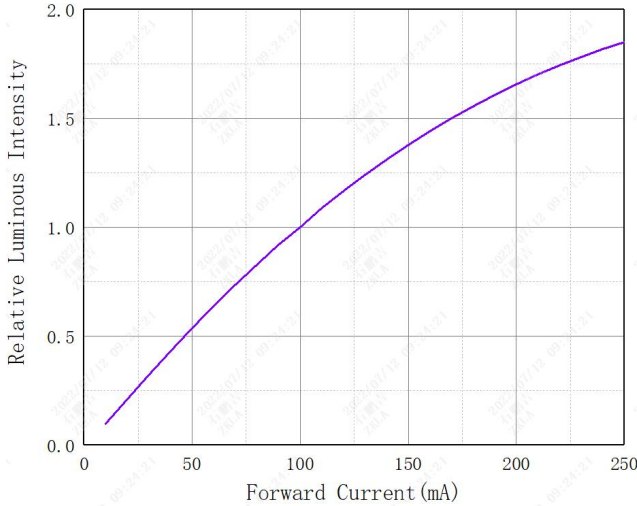
正向电流与辐射通量曲线图
